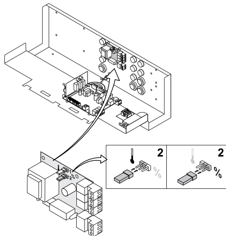
Bild 10 Jumper 2 umstellen
