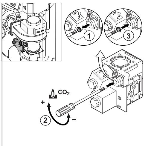
Bild 21 Einstellen Mindestleistung 200-5 und 200-6 Kessel
