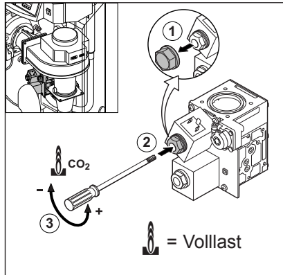
Bild 20 Einstellen Volllast
