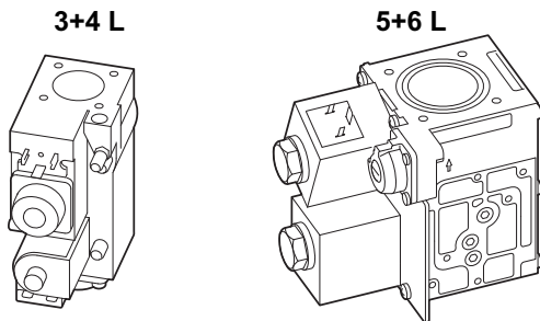
Bild 04 Gasarmaturen
