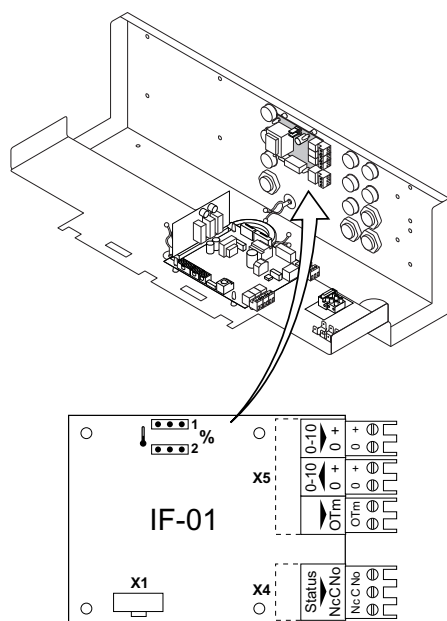
Bild 09 Optionale Steuerungsplatine 0 - 10 V (IF-01)
