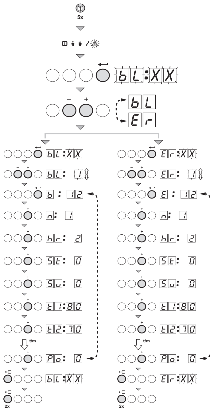
Bild 29 Aufruf von Blockierungen oder Störungen
