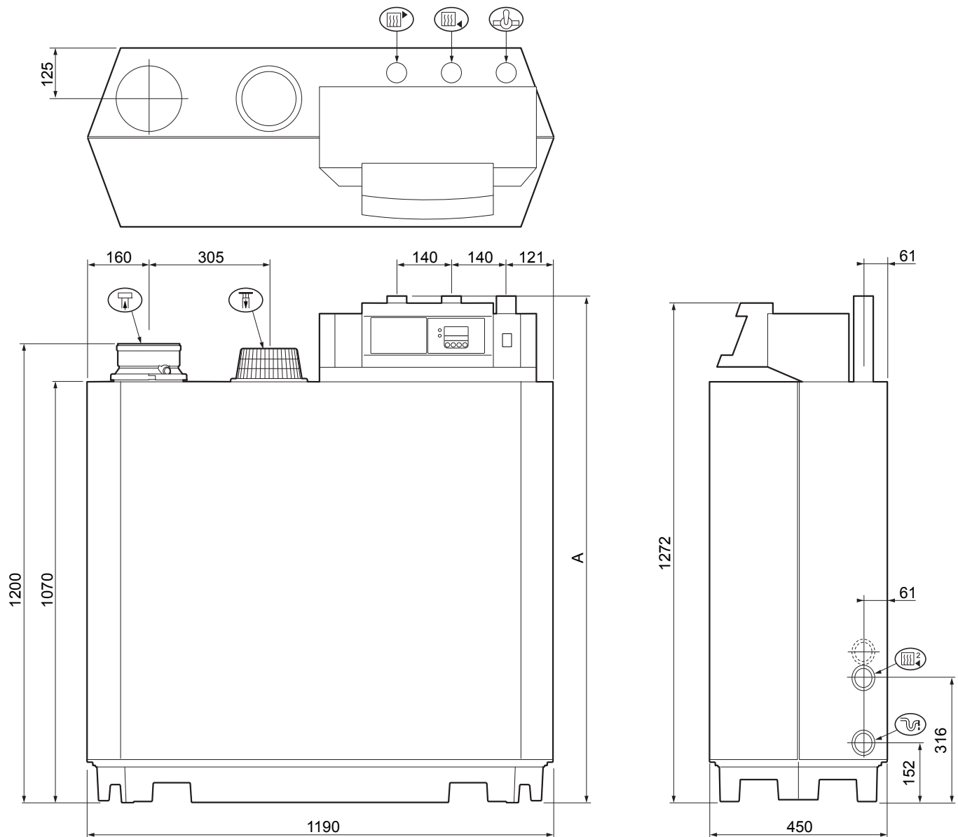
Bild 01 Ansichtszeichnungen
