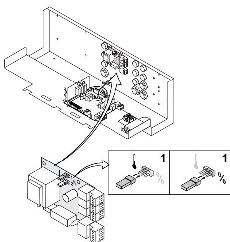
Bild 11 Jumper 1 umstellen
