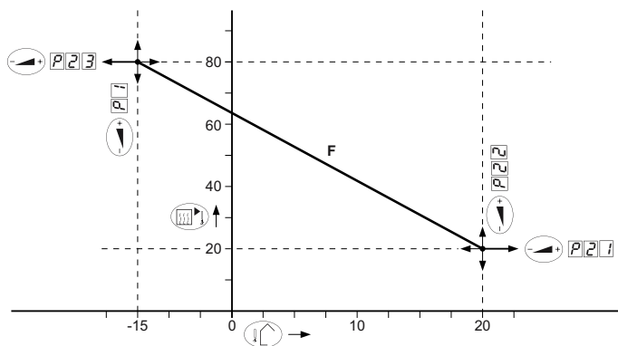
Bild 13 Heizkurve
