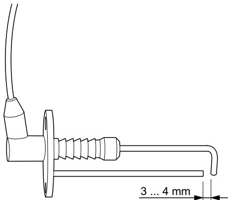
Bild 28 Kontrolle der Zündelektrode
