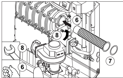
Bild 27 Reinigung des Brenners
