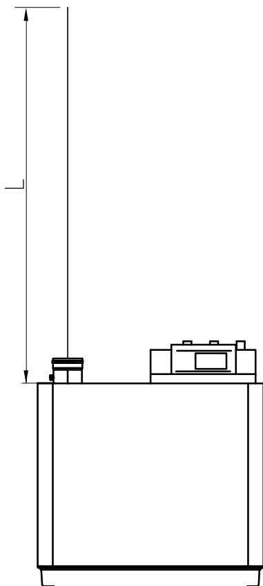
Bild 05 Leitungsverlauf bei Raumluftabhängigem Betrieb
