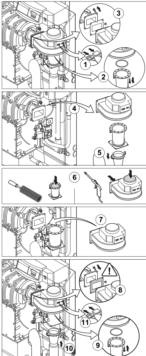
Bild 25 Reinigung des Gebläses 200-5 und 200-6 Kessel
