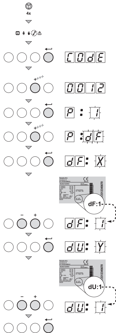
Bild 18 Wiederherstellen von Werkseinstellungen
