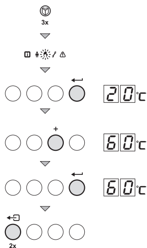
Bild 19 Einstellen des Handbetriebs
