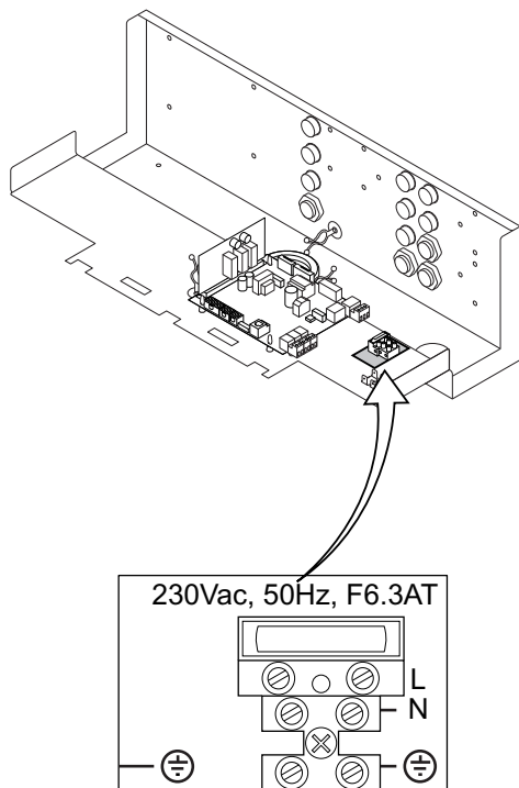
Bild 06 Netzkabel anschliessen
