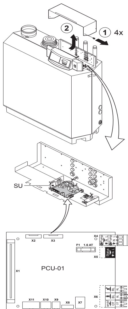
Bild 07 Standard-Steuerplatine (PCU-01)
