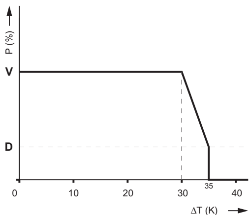
Bild 03 Charakteristik der Leistungsregelung
