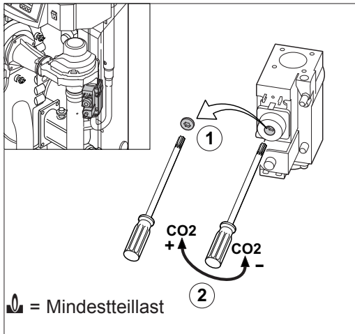
Bild 22 Einstellen Mindestteillast 200-3 und 200-4 Kessel (nur Mindestteillast)
