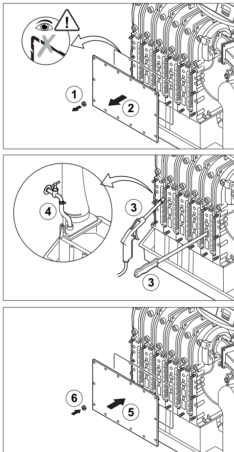
Bild 26 Reinigung des Wärmetauschers
