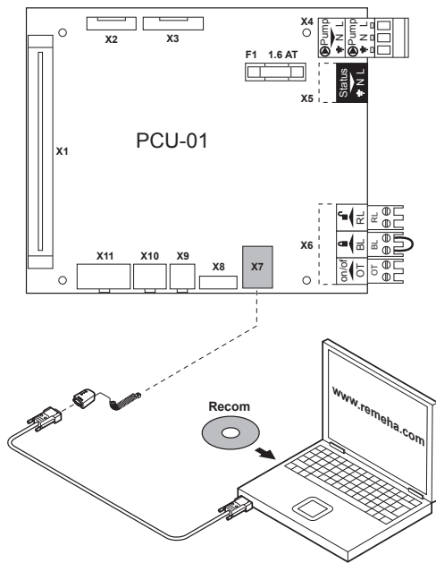
Bild 08 Anschluss PC
