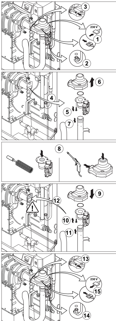
Bild 24 Reinigung des Gebläses 200-3 und 200-4 Kessel
