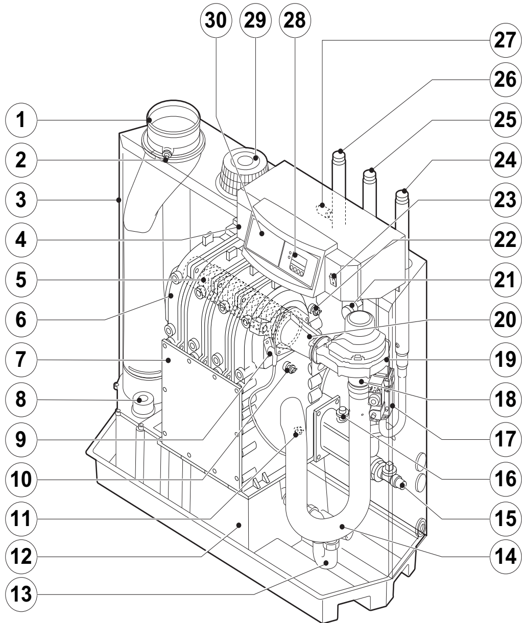
Bild 33 Querschnitt (abgebildet ist die 200-5 Ausführung)
