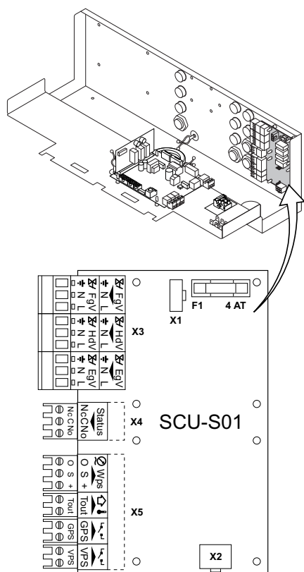
Bild 12 Erweiterte Steuerungs-/Sicherheitsplatine (SCU-S01)
