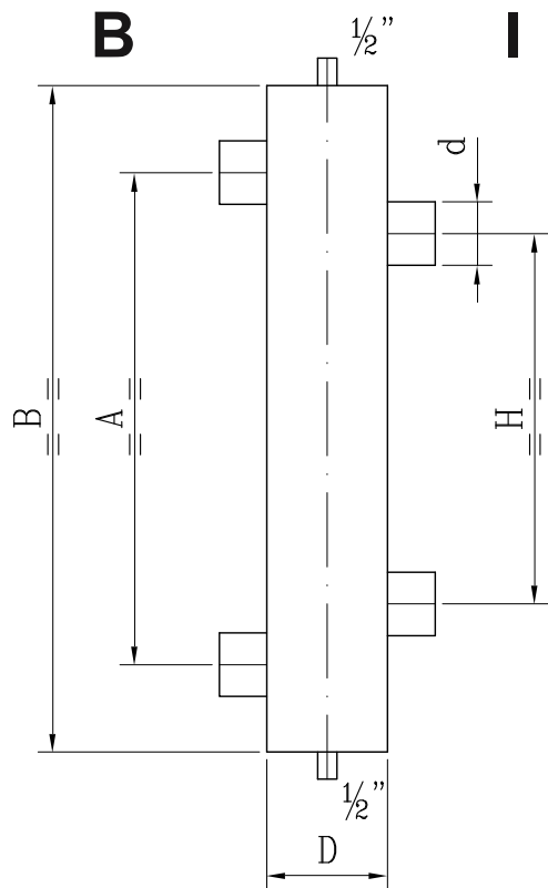
Bild 35 Hydraulische Weiche
