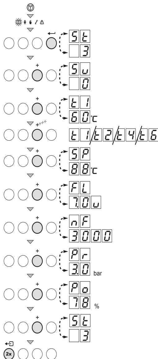
Bild 15 Anzeige aktueller Werte
