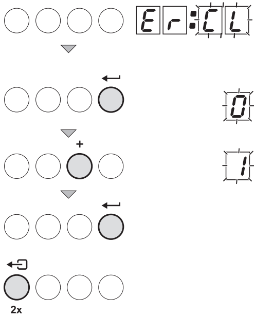
Bild 30 Löschen von Störungen
